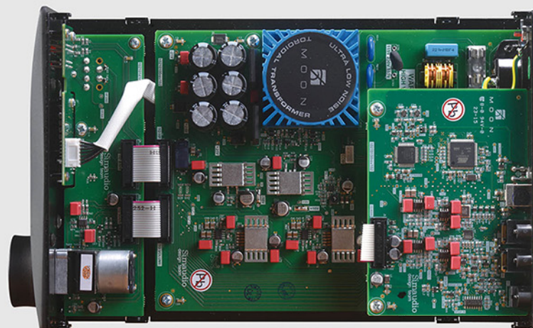
内部结构为模块化设计，DAC、模拟放大和控制各有独立线路板
